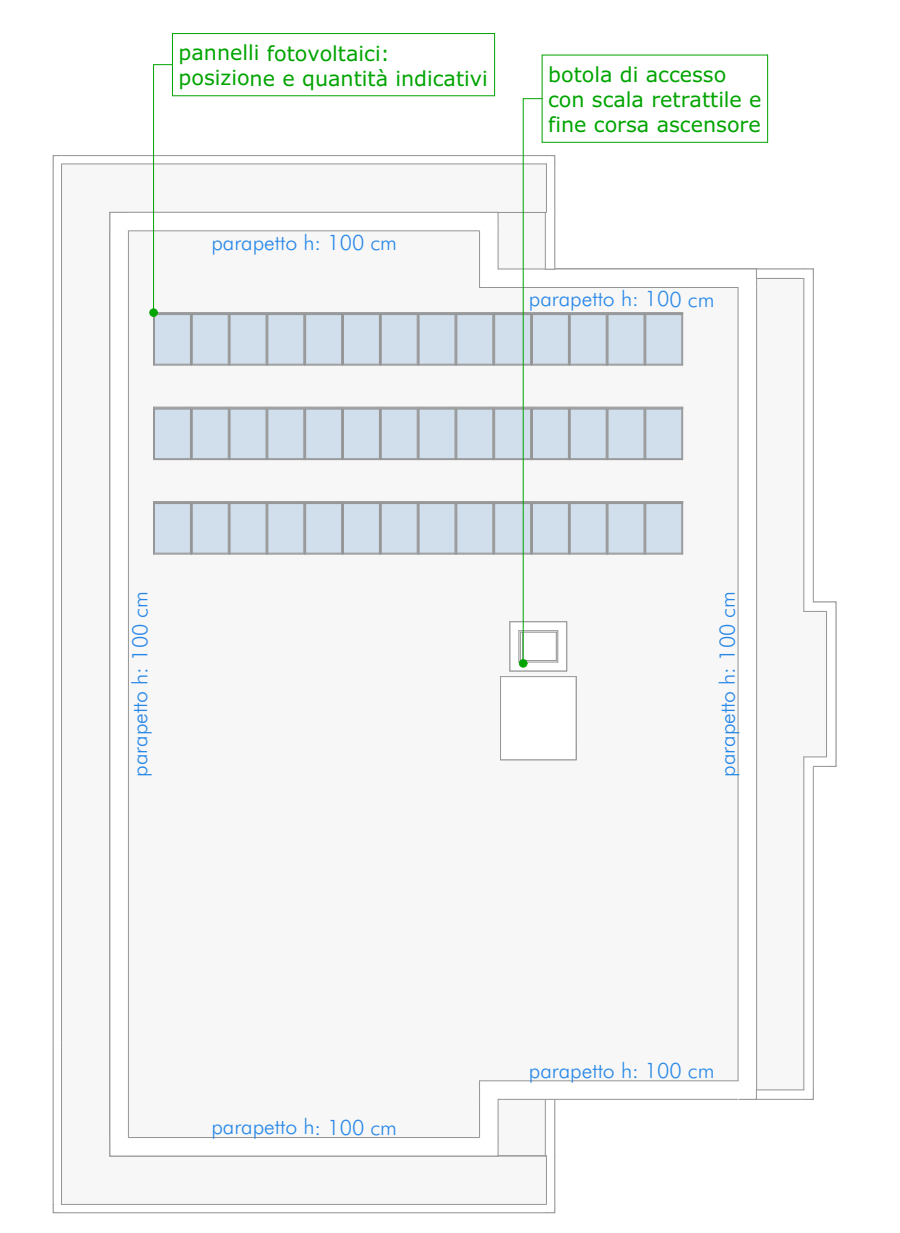
3. Piano Copertura A 1:200
