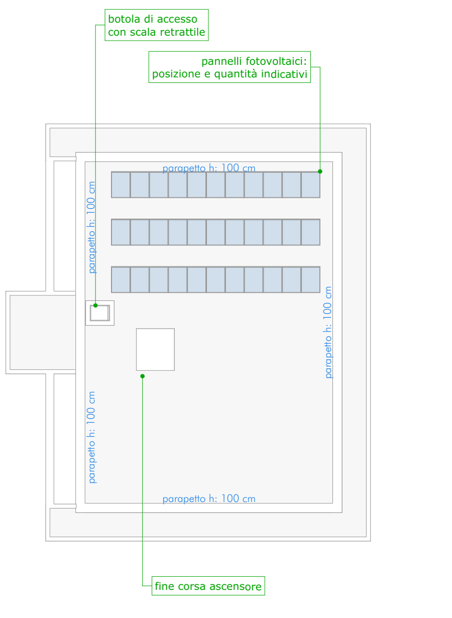
3. Piano Copertura B 1:200
